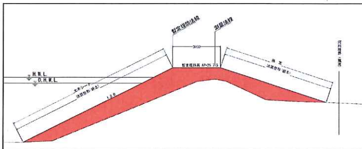
I期施工の断面図
