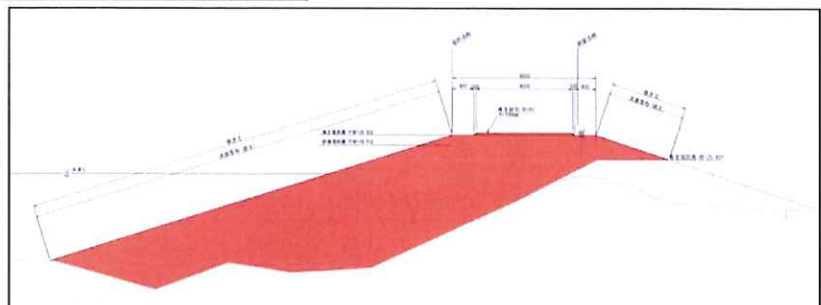
II期施工の断面図
